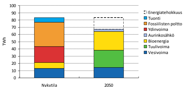
Kuva 2. Energiantuotantopaletin uudistuminen.
